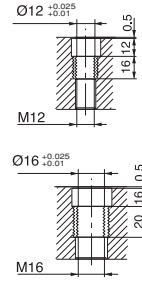
Çelik burçlu Referans Nr. 2575 Steel bush Reference No. 2575
